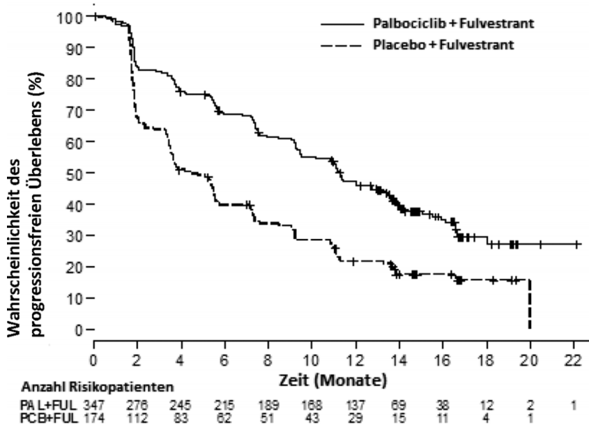
Abbildung 2. Kaplan-Meier-Plot des progressionsfreien Überlebens (Prüfarzt-Bewertung, Intent-to-treat-Population) – PALOMA-3-Studie
