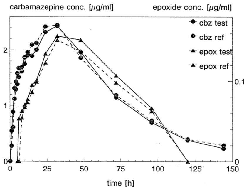
Mittlere Serumspiegelverläufe im Vergleich zu einem Referenzpräparat in einem Konzentrations-Zeit-Diagramm.
